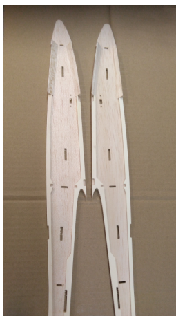
Slepené bočnice včetně trojúhelníkových listů (předek trupu)
